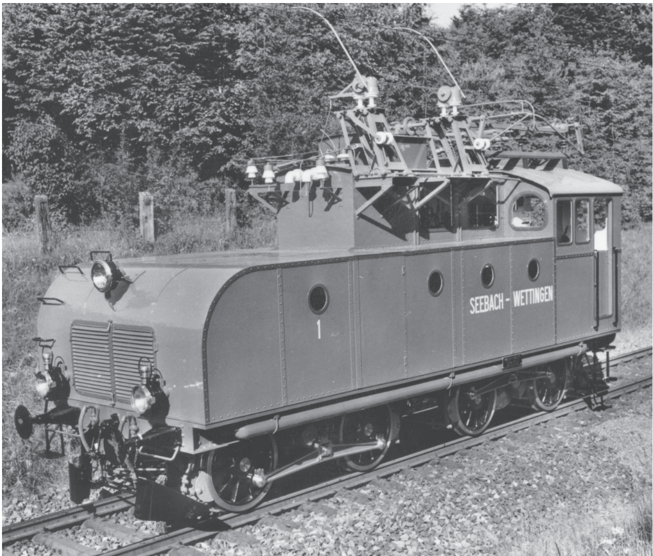
Elektrolok Ce 4/4 Nr. 1 Eva, Einphasenwechselstrom-Lokomotive der MFO. Versuchslokomotive Seebach-Wettingen. Baujahr 1904. Bild: Verkehrshaus der Schweiz, Luzern
